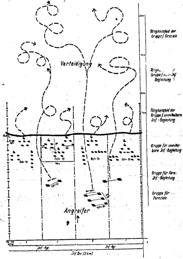
Schematische Darstellung des Kampfwageneinsatzes im Angriffsstreifen einer Inf.-Div.
