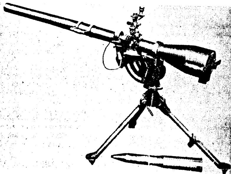
75 m/m rekylfri kanon. Vikt 50 kg, granaten 9 kg. 5 mans betjäning Skottvidd över 6 km. Kan bäras i all slags terräng. (En 75 m/m fältkanon drages av 6 hästar!)
